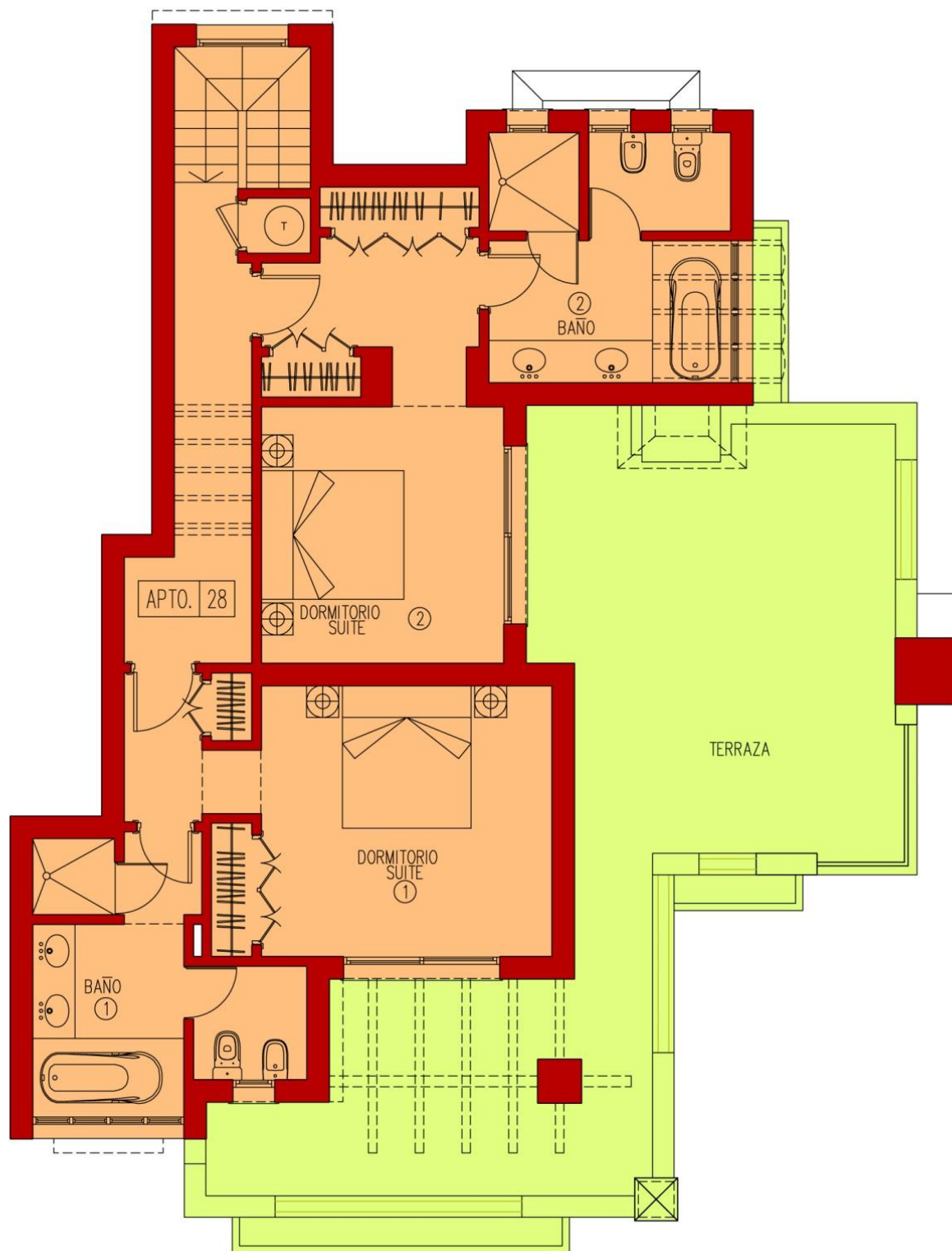
PLANTA SEGUNDA
